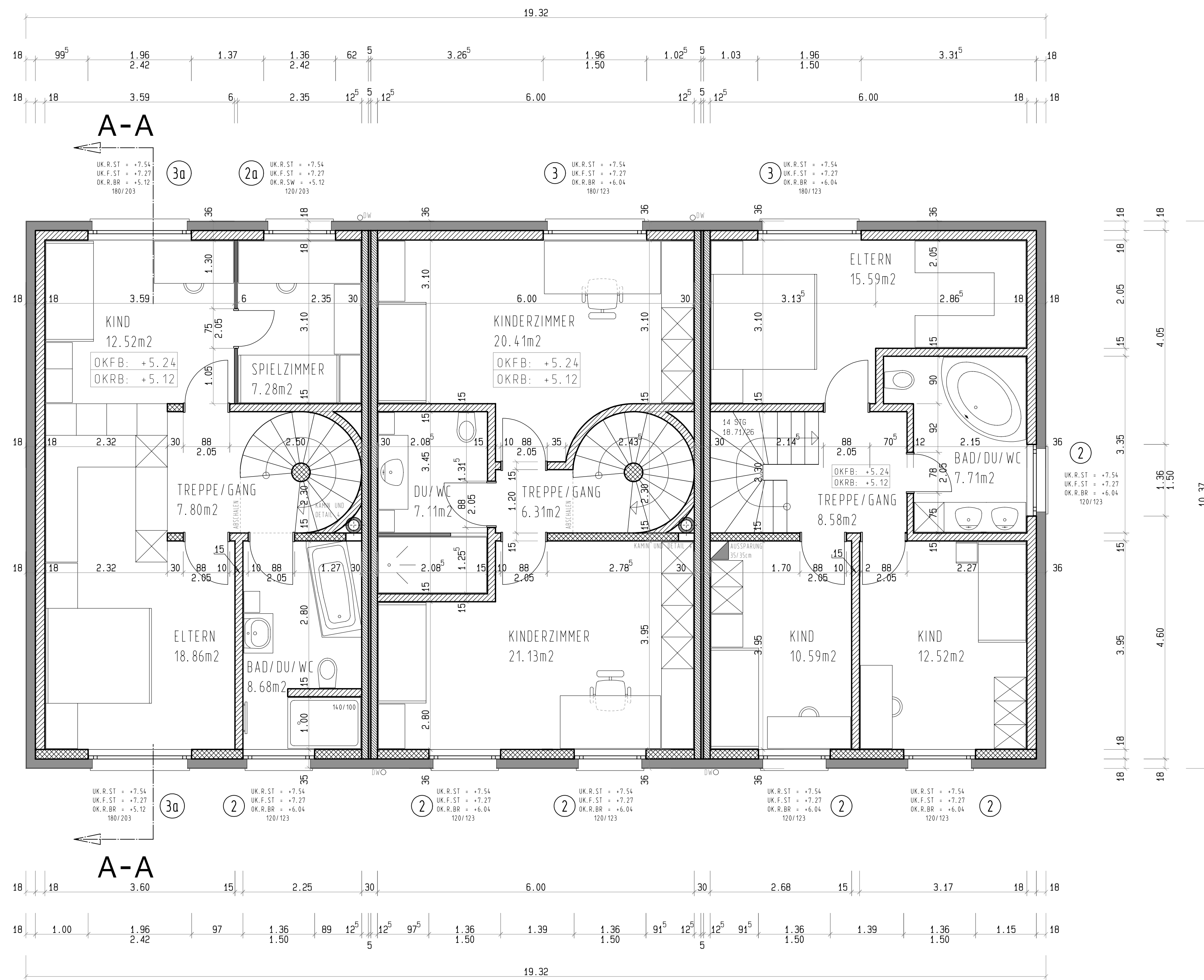
HAUS 1 HAUS 2 HAUS 3 2.OBERGESCHOSS 1:50
