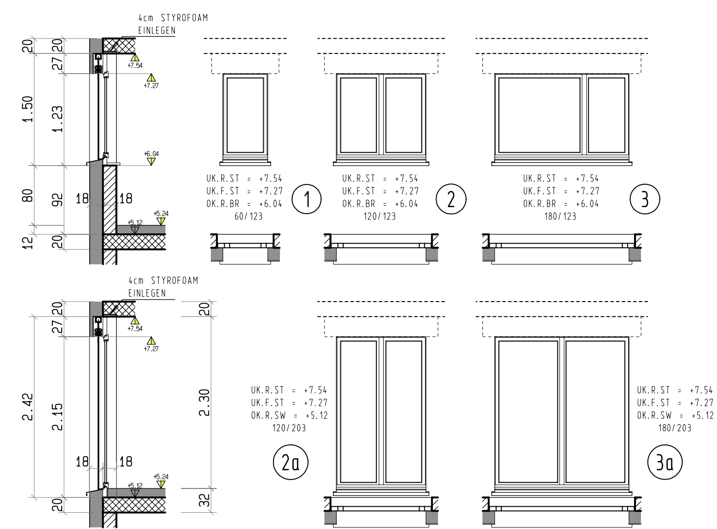
WERKPLAN 1:50
