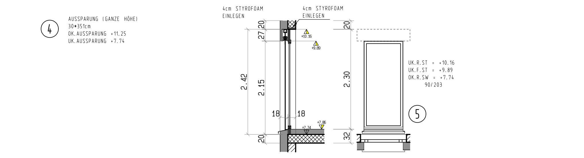
WERKPLAN 1:50
