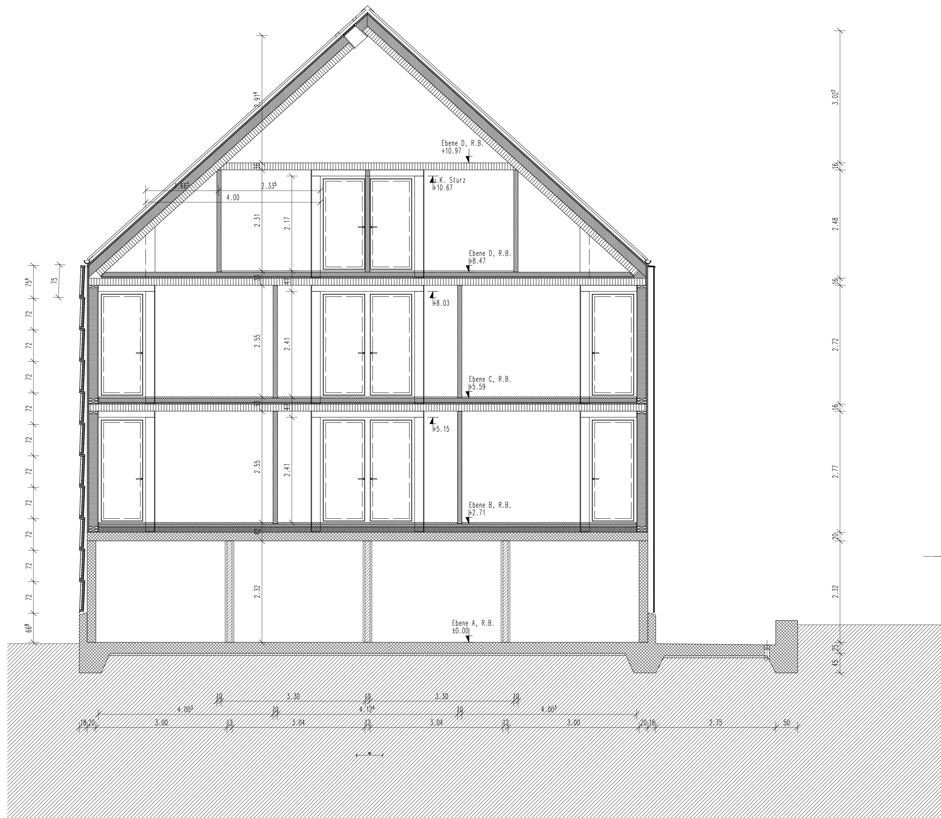
Schnitt P-P
