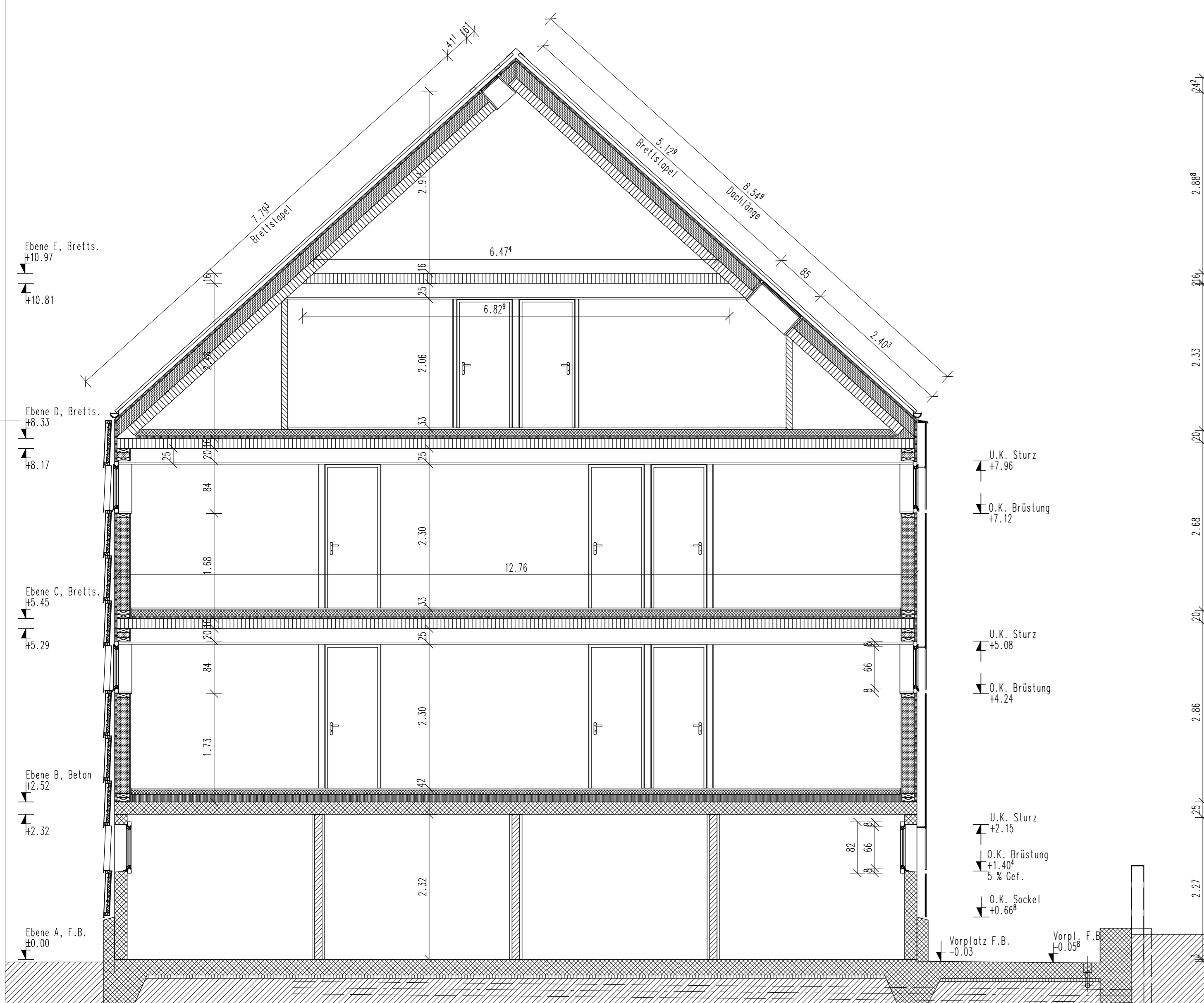
Schnitt Q-Q
